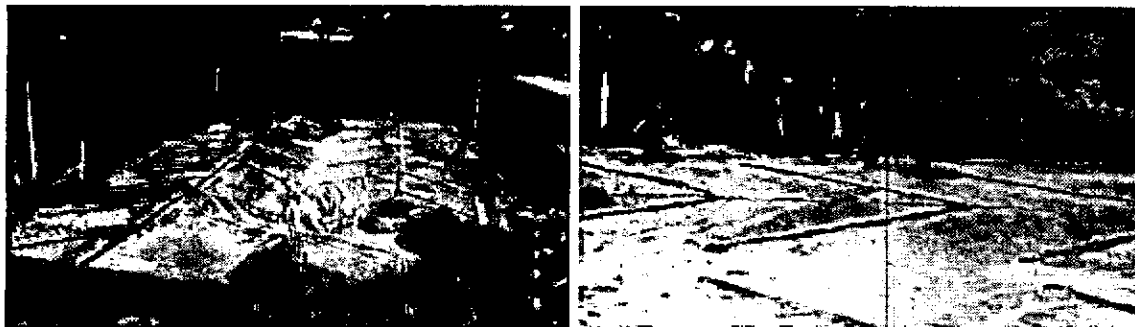
Foto 3 y 4. Problemática de saturación del suelo en la construcción de la cancha de fútbol sintética en Betania. Levantó. Juan David González Orozco – Profesional Universitario.
